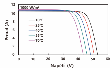
I-V Charakteristiky za různých teplot
