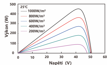
P-V Charakteristiky za různého osvitu
