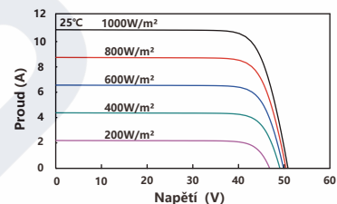
I-V Charakteristiky za různého osvitu
